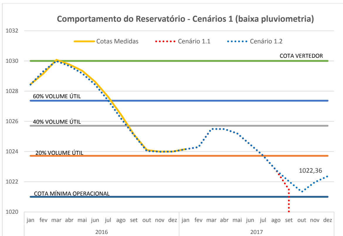
Gráfico 6: Comportamento do reservatório – cenários 1.1 e 1.2 (acionamento de 12,1% até junho e 30% de julho a dezembro).
